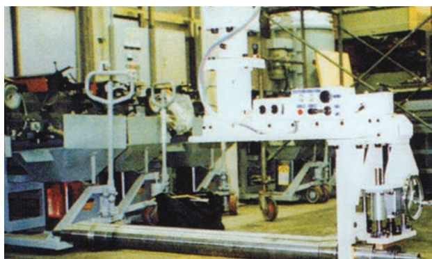
シャフト装着作業 Shaft mounting operation
