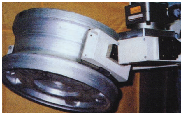
外径クランプ・反転作業 Outer diameter clamp inversion work
